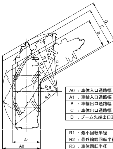
4輪ステアリングで右折する場合
